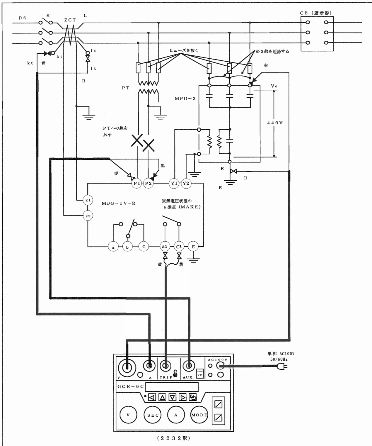
【図 方向地絡継電器の試験 [三菱電機MDG-1V-Rの場合]】
