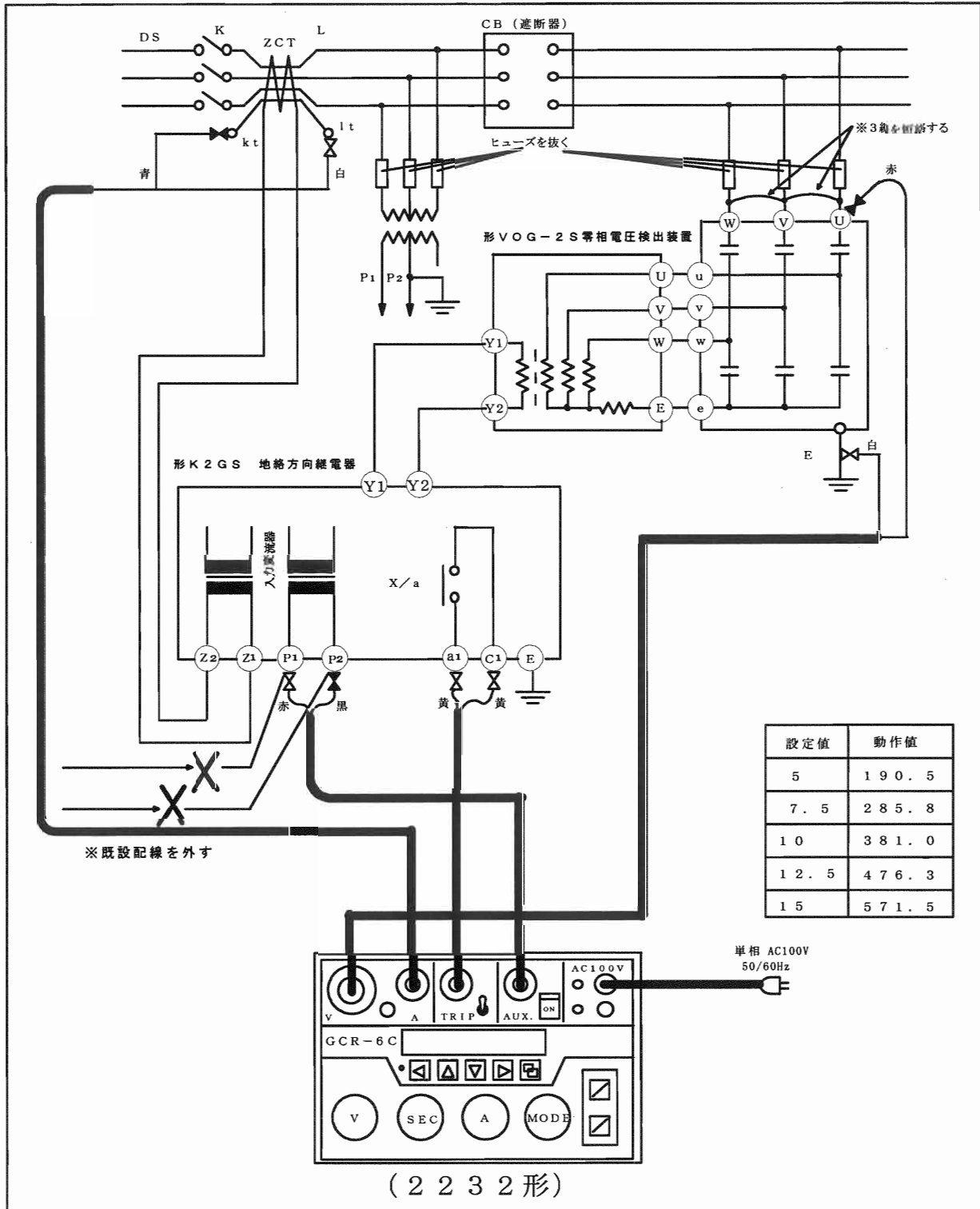
【図 方向地絡継電器の試験 [オムロンK2GS, VOG-2Sの場合]】
