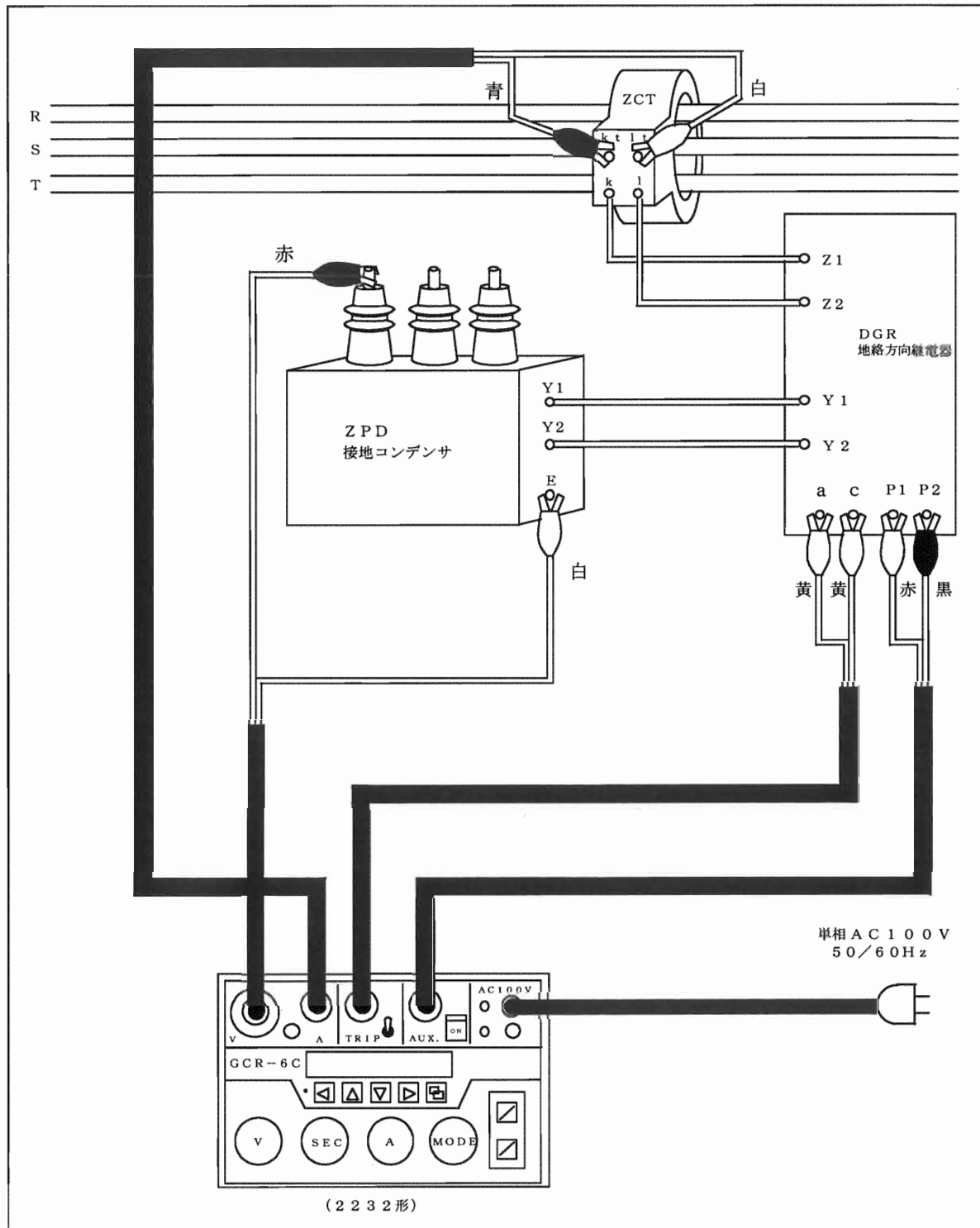
【図 地絡方向継電器（DGR）と2232の結線】
