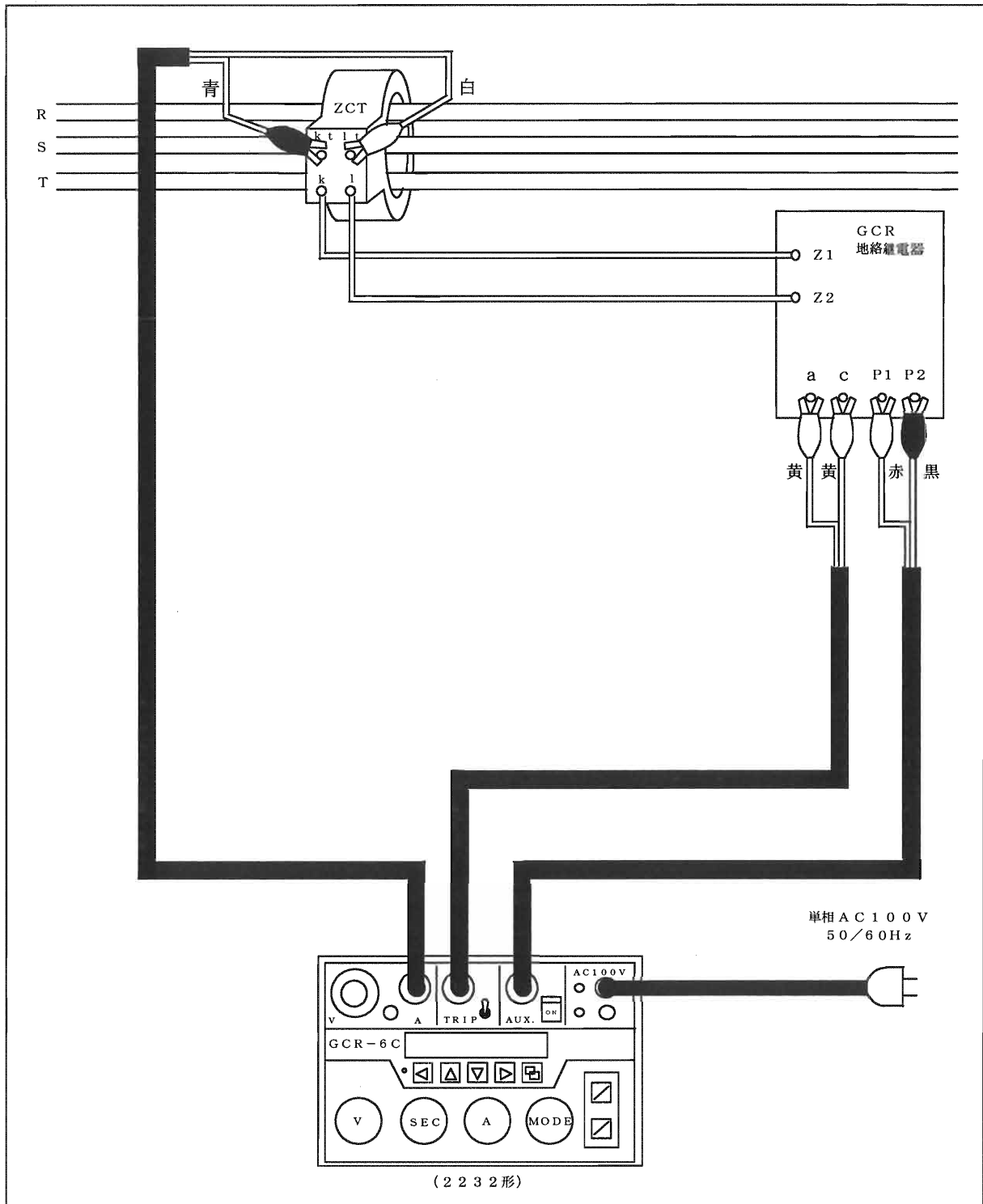
【図 地絡継電器 (GCR) と 2232 の結線】
