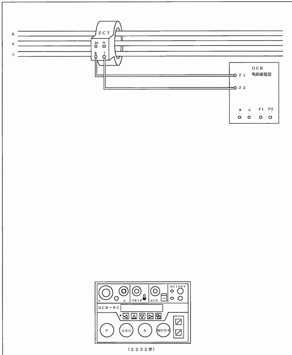
【図 地絡継電器（GCR）と2232の配置】
