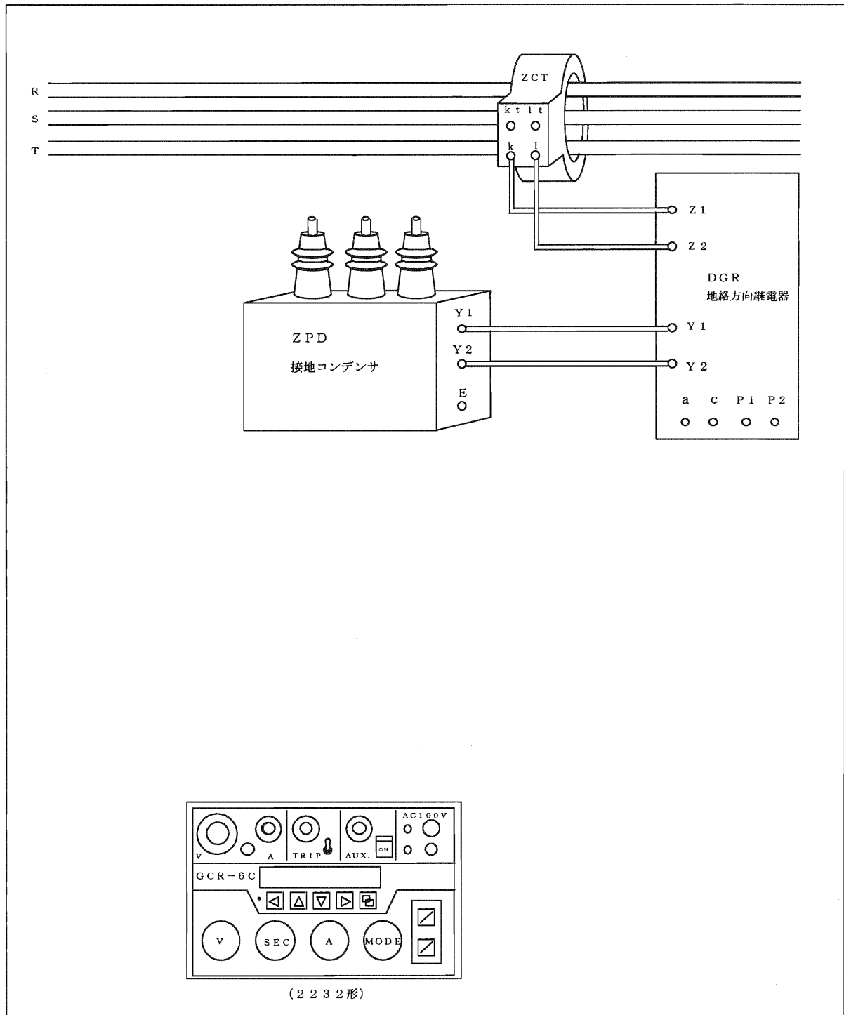
【図 地絡方向継電器（DGR）と2232の配置】
