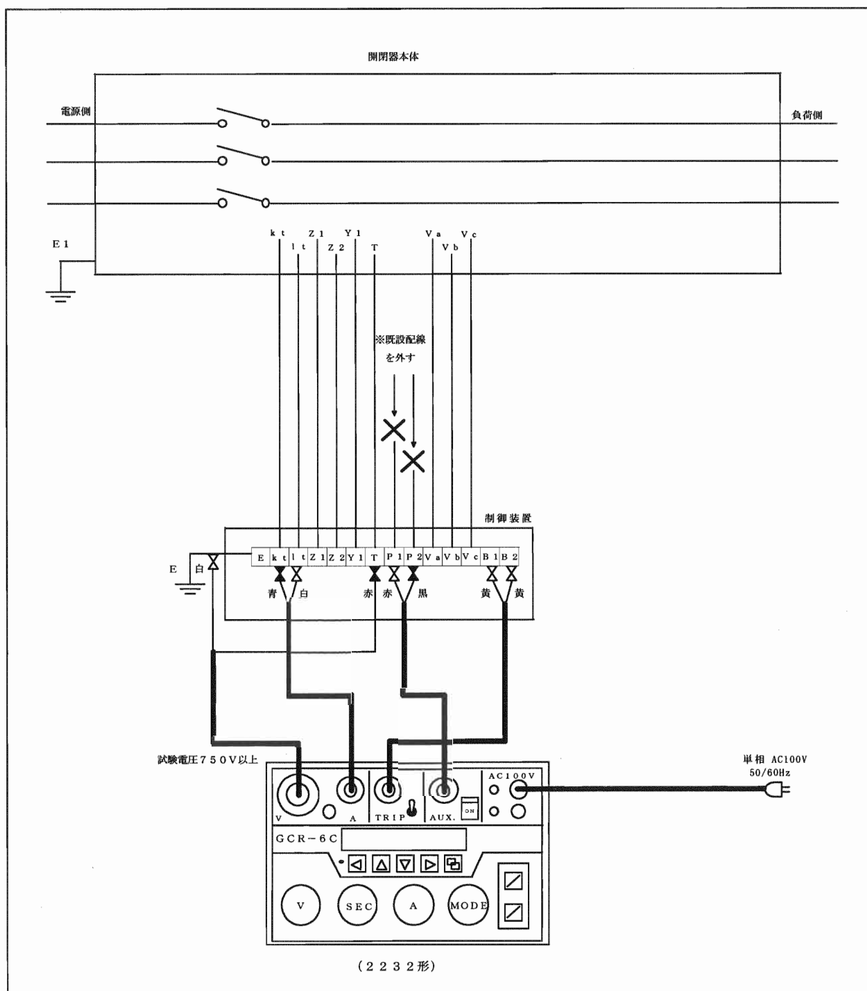
【図 方向地絡継電器の試験 [エネルギーサポートCLD-R DGR付PASの場合]】
