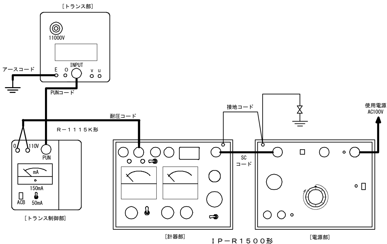
図2 試験器結線図
