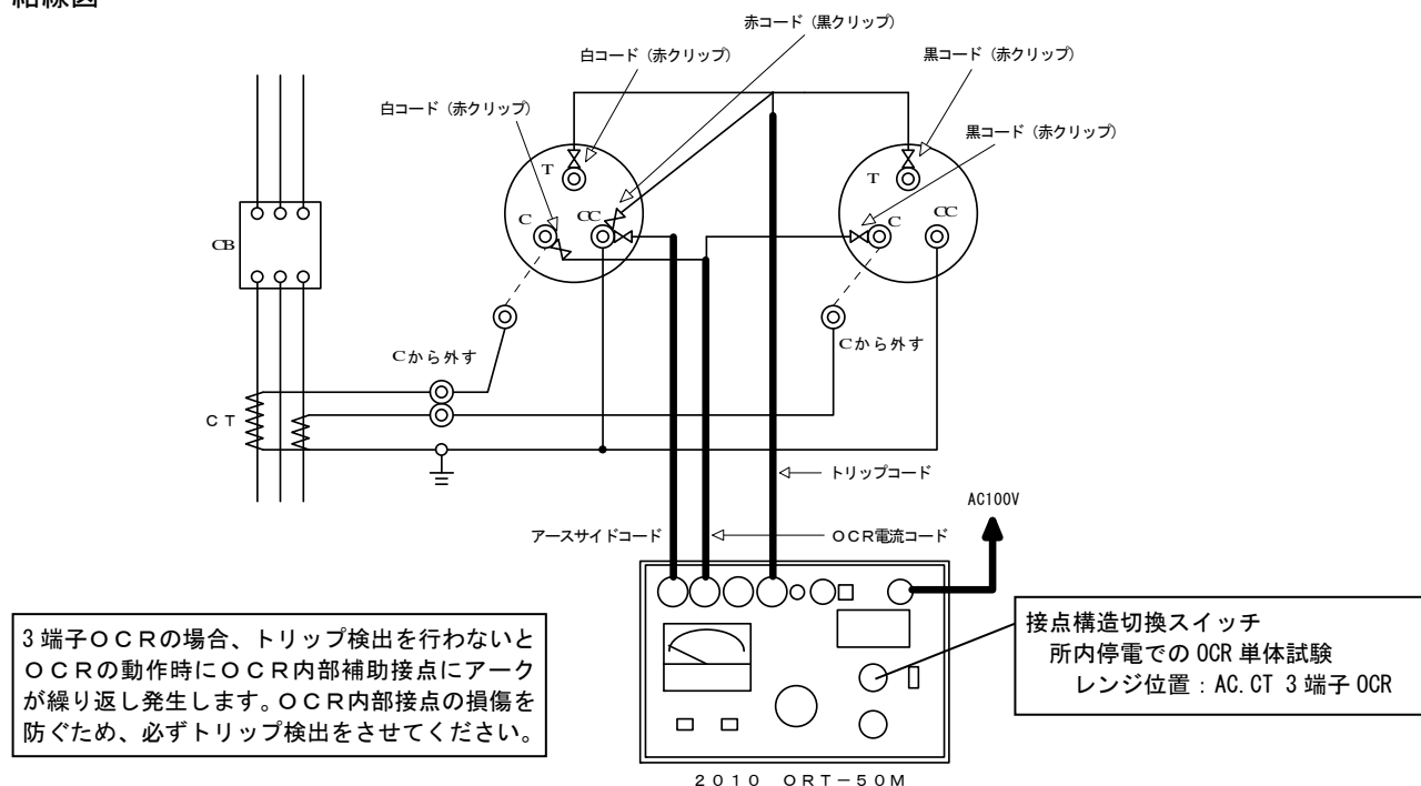
結線図
