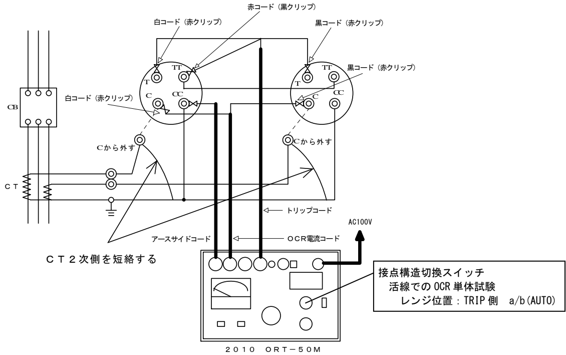
図 17 限時要素の動作電流特性試験
