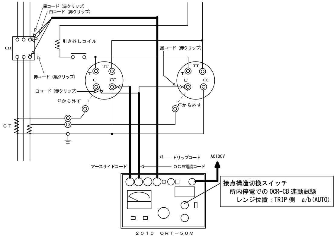
図 2 2 CB連動での限時要素動作時間試験
