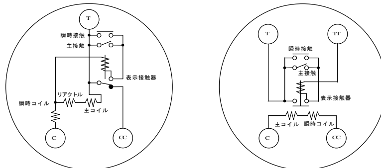
電流引き外し方式：3端子OCR 電圧引き外し方式：4端子OCR 過電流継電器試験の内部回路例
