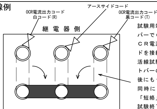
C T 側 高圧受電盤試験用端子の結線例
