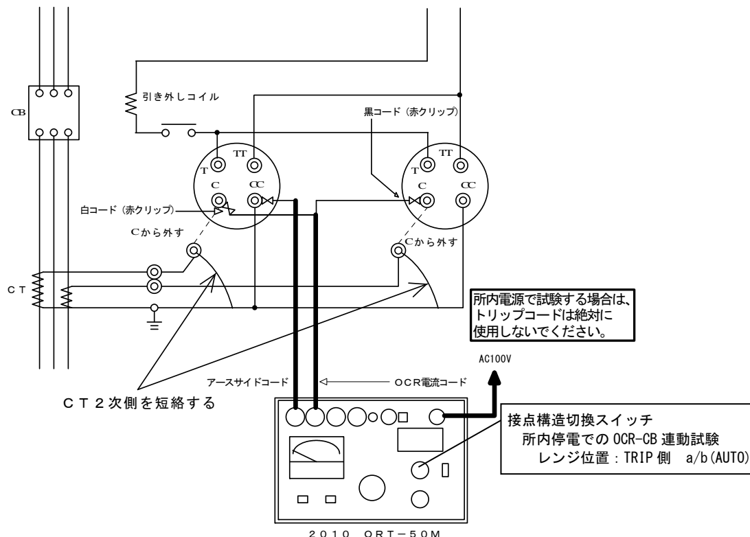
図 2 8 CB連動での瞬時要素動作時間試験
