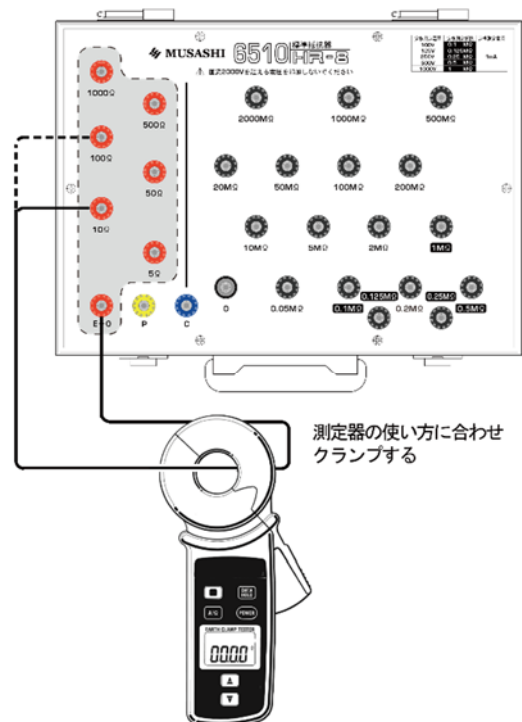
【クランプタイプ接地抵抗計での接続】
