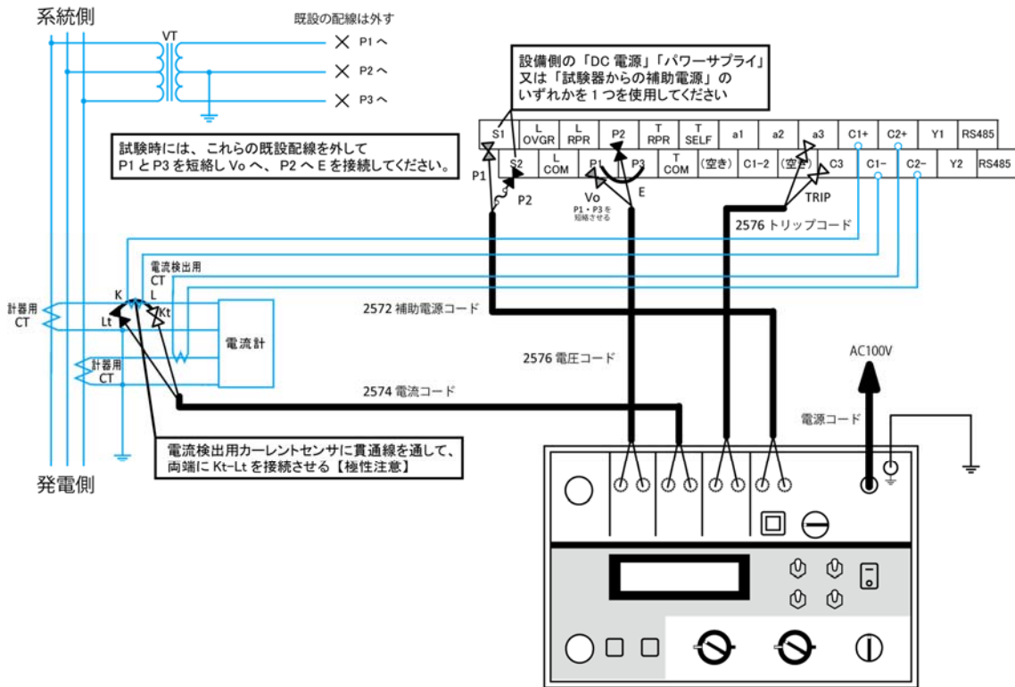
図 2 逆電力継電器の配線例
