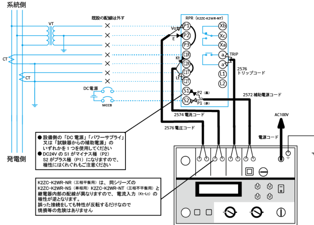
図 2 逆電力継電器の配線例《オムロン製 K2ZC-K2WR-NT》
