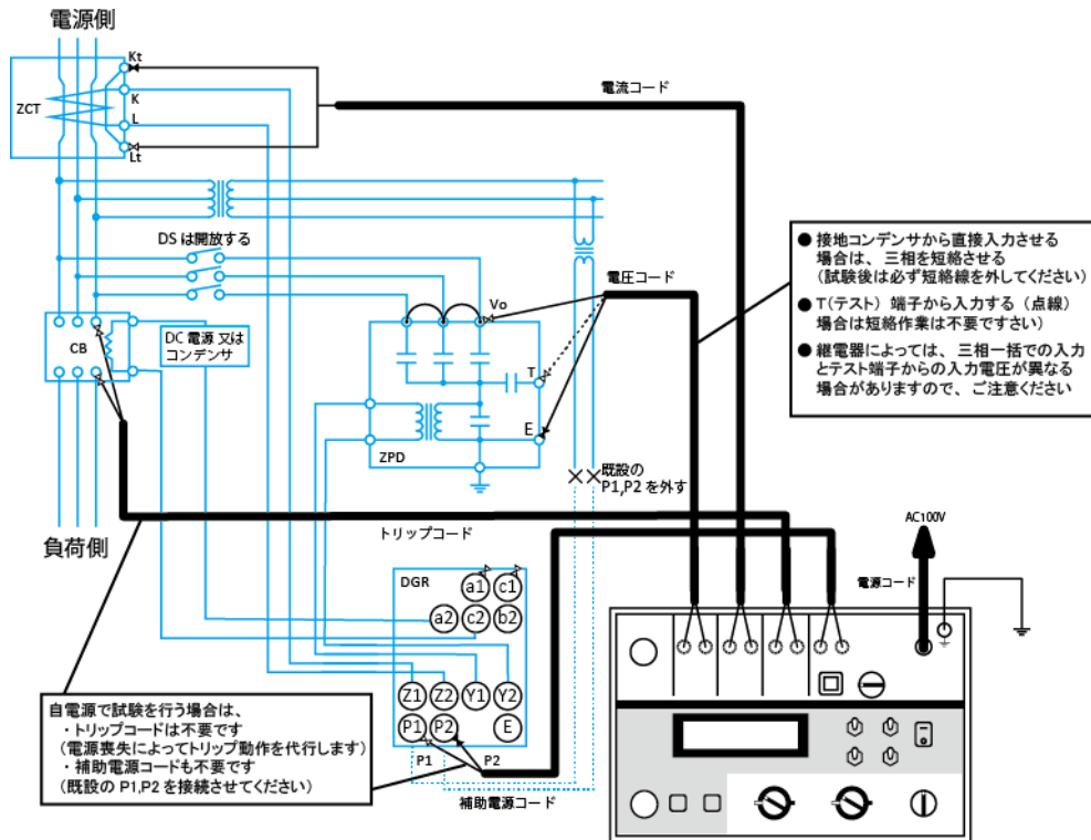
図2 CB連動試験の結線
