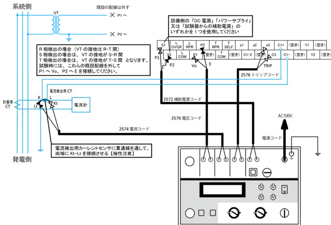
図1 逆電力継電器の配線例
