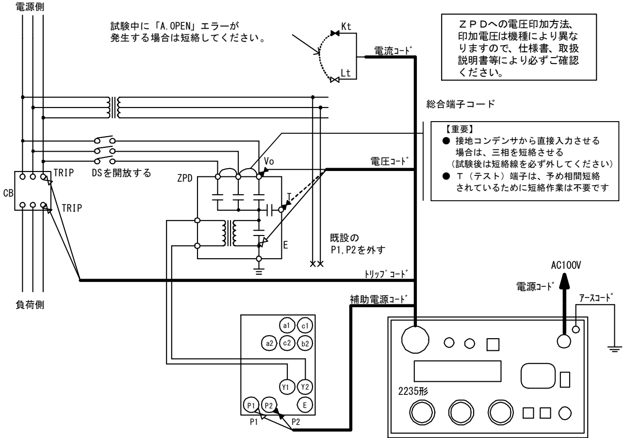
図 2 CB連動試験の結線
