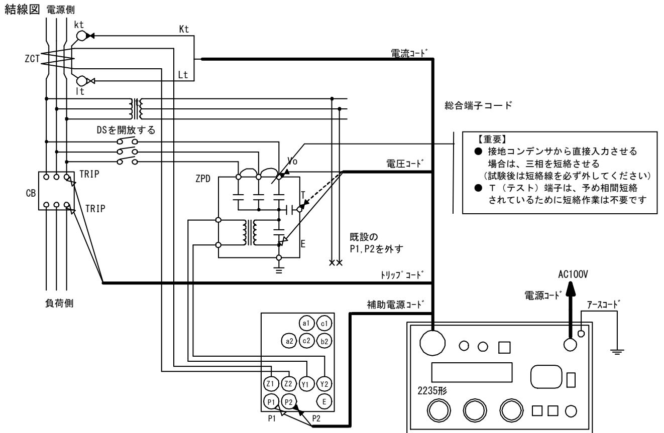
図2 CB連動試験の結線
